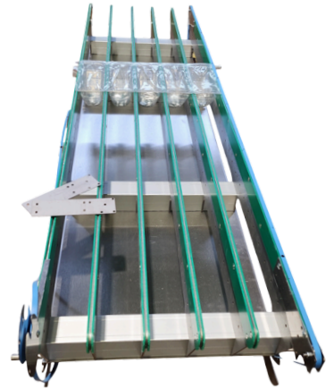
Nastro trasportatore per tramezzini
