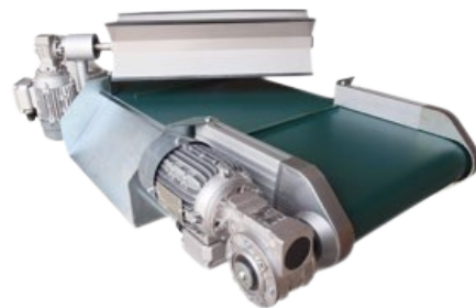
Separatore a palette
