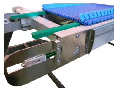
Sostegno tela modulare con sistema di tiro
