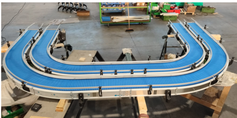
Nastro a a ferro di cavallo per collegamento confezionatrici
