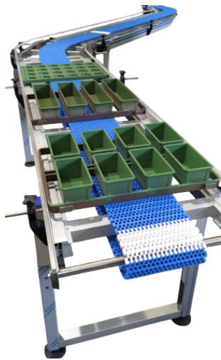
Sistema di trasporto per pane in cassetta
