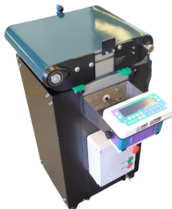
Nastro pesato per controllo peso di sacchetti provenienti da confezionatrice automatica
