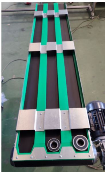
Nastro piano asservimento cobot montaggio cuscinetti
