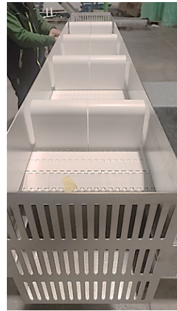
Nastro in AISI 316 per trasporto patate
