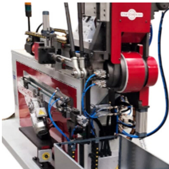
Nastro piano In AISI 1200x40mm-Tela PU Verde integrato in Macchina piega tubi
