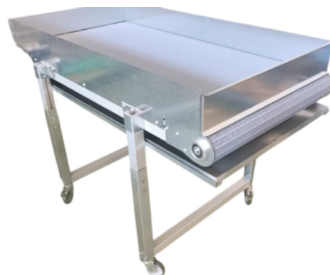
Nastro in tapparella modulare con Leccarda
