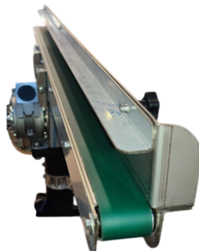
Nastro piano In AISI 1200x40mm-Tela PU Verde integrato in Macchina piega tubi
